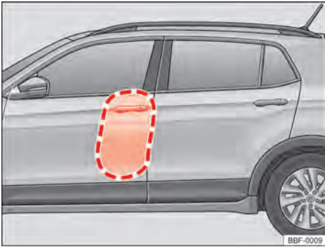
Fig. 36 Del lado izquierdo del vehículo: áreas de expansión del airbag lateral.
