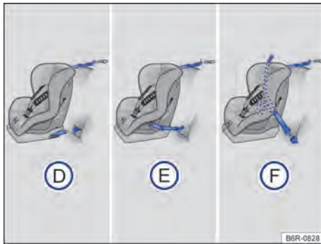
Fig. 40 En el asiento trasero: las figuras D y E muestran el principio de fijación del sistema de retención infantil en los ojales de retención inferiores y con el cinturón de fijación superior. La figura F muestra la fijación del sistema de retención para niños con el cinturón de seguridad del vehículo y con el cinturón de fijación superior.
