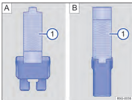
Fig. 162 Retirar o colocar el fusible con la pinza de plástico: A fusible plano, B : fusible de bloqueo.
